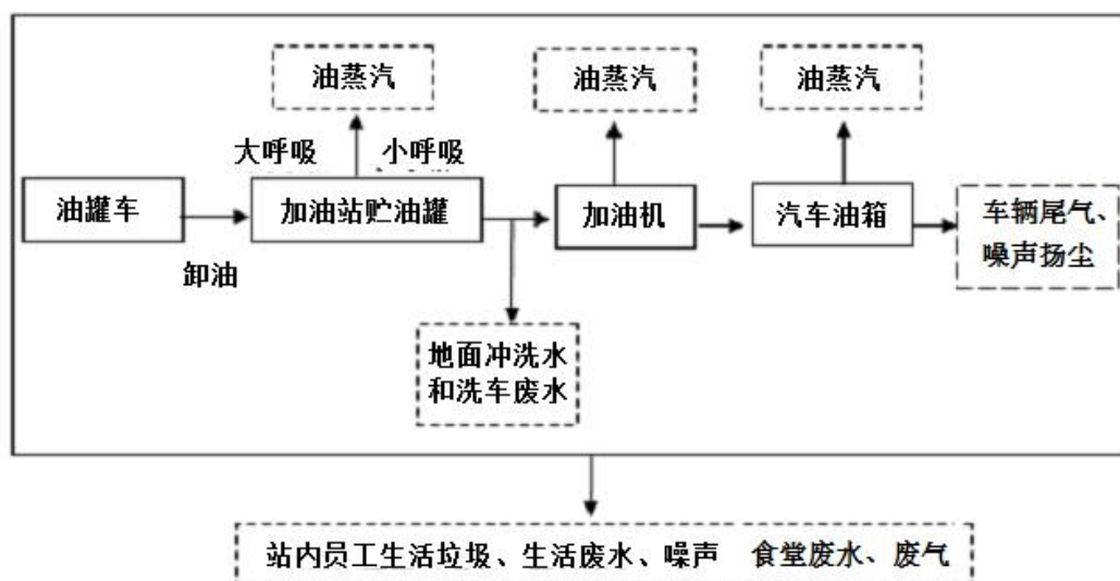
图 3-1 运营期工艺流程和产污节点图
